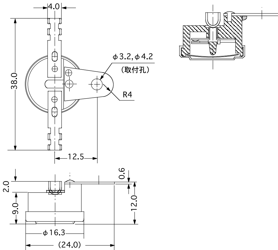
外形寸法図 TH-51WF171 型
